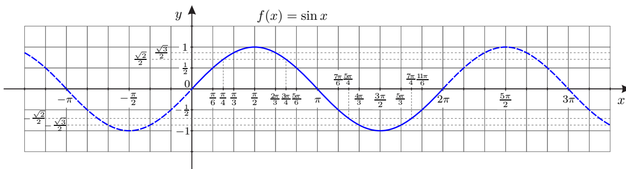
Funkcja sinus: f(x) = \sin x
