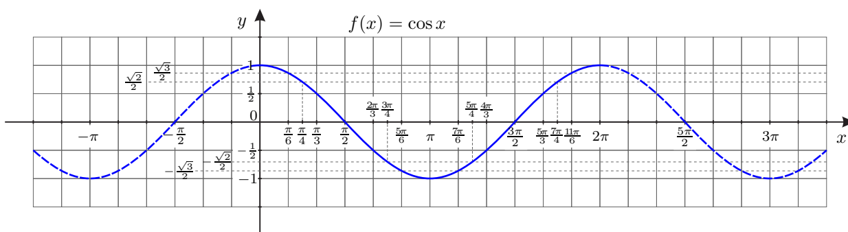
Funkcja cosinus: f(x) = \cos x
